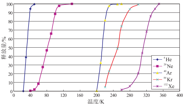
图 1 稀有气体低温富集分离实验结果
