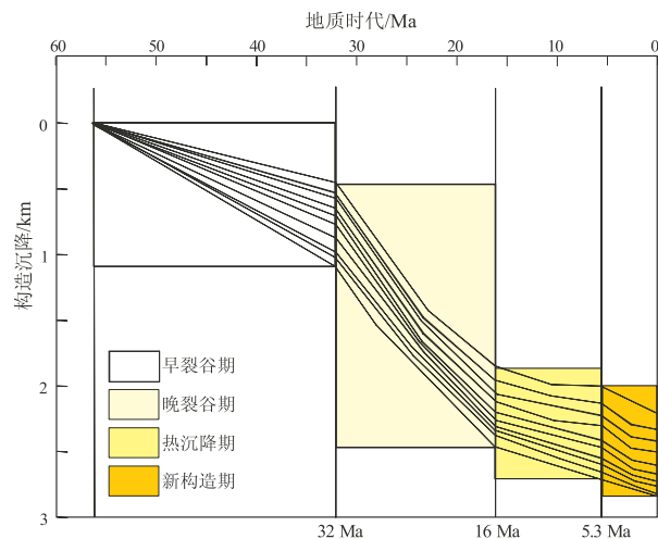
图 3 琼东南盆地构造沉降史曲线
