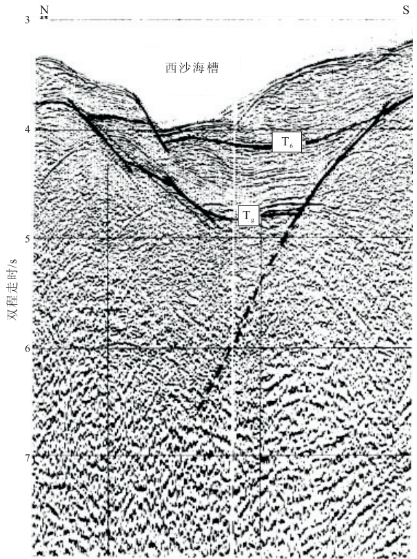
图2 过西沙海槽南北向广角地震探测剖面
