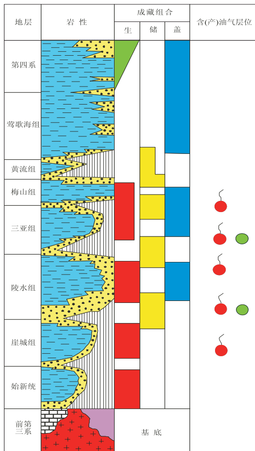
图 5 琼东南盆地主要生储盖组合示意
