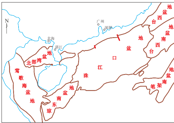
图1 南海北部陆坡主要沉积盆地的分布特征
